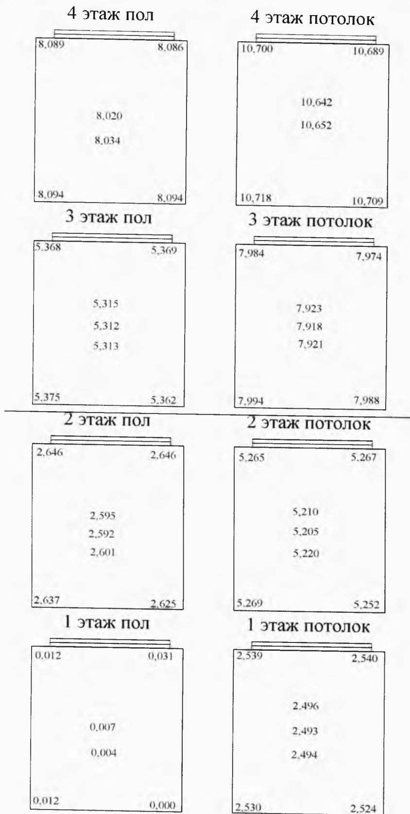
Рисунке №4. Прогибы панелей перекрытия.
