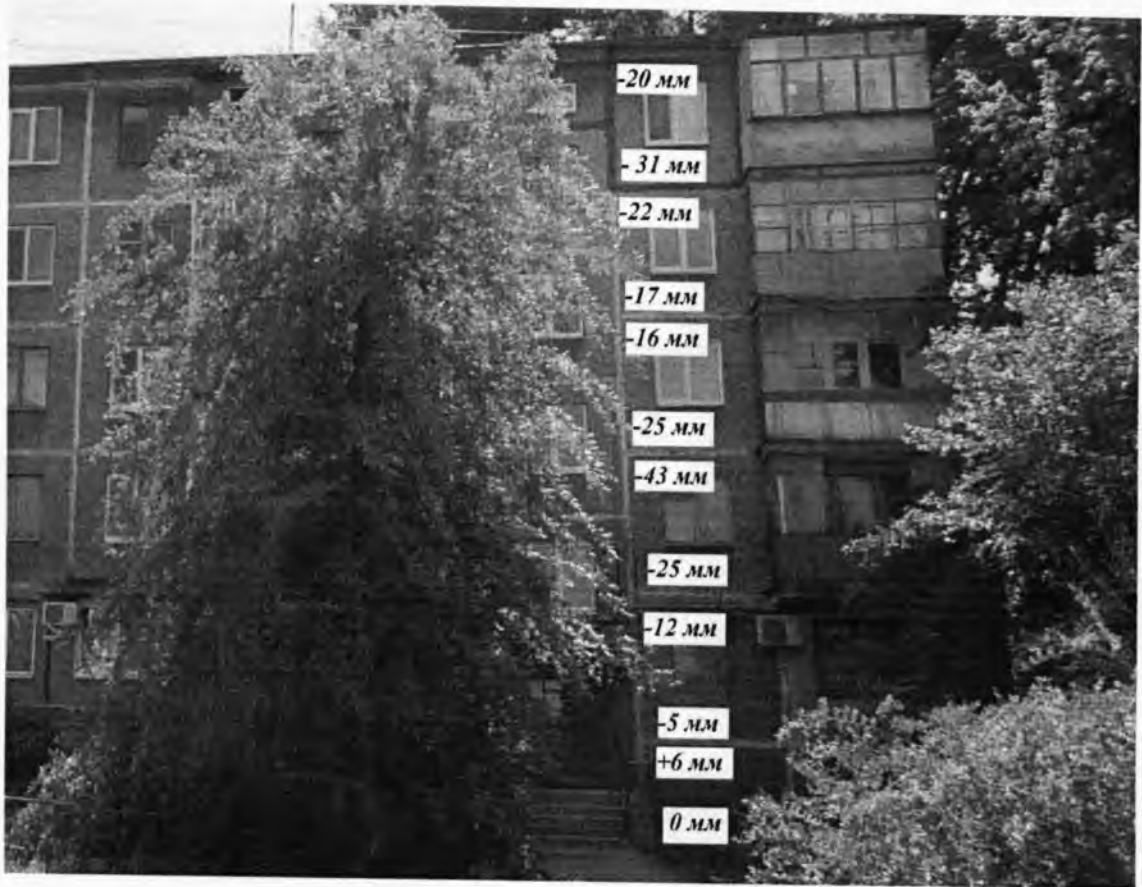
Рисунке №5. Измерения вертикального отклонения фасада здания.
